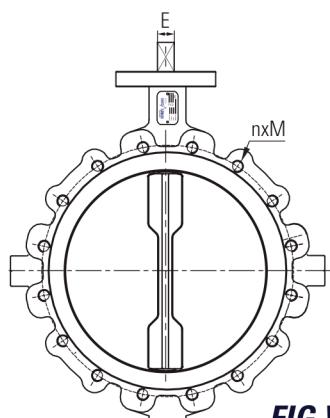
FIG V109 Lug Type
